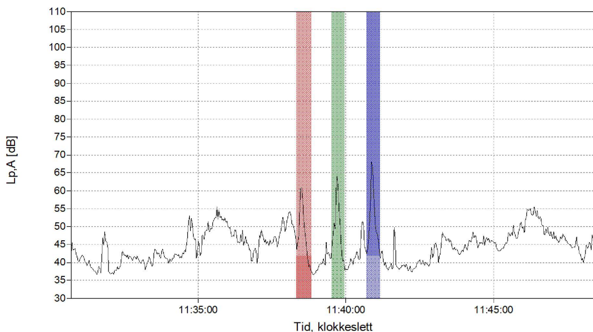
Figur 1 Målt A-veid ekvivalent lydtryknivå, L_{p,A} pr. sekund for de tre kjøretøypasseringene på Vålerbanen 4. juni 2019.
